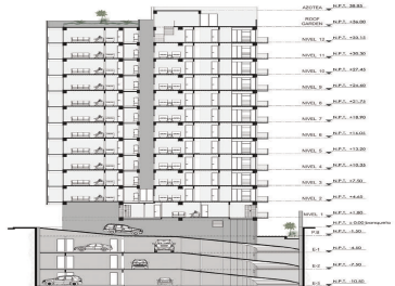
CORTE LONGITUDINAL
