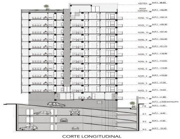
CORTE LONGITUDINAL
