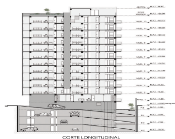
CORTE LONGITUDINAL
