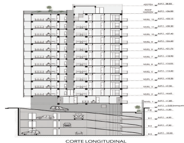
CORTE LONGITUDINAL
