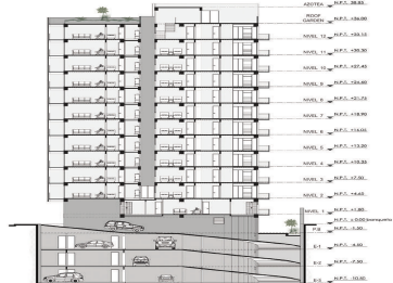
CORTE LONGITUDINAL
