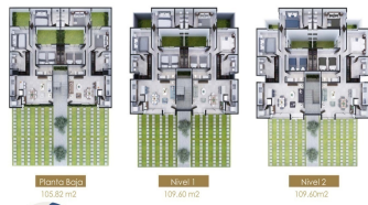
Planta Sola
