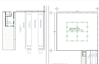
- PLANO ARQUITECTÓNICO-
