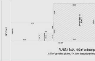
Bodega Santa Rosa Jáuregui, plano planta baja
