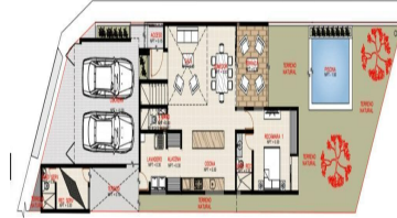
PLANTA BAJA
