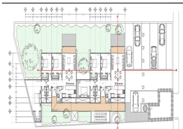
PLANTA ARQUITECTONICA SERVIDOR NIVEL + 0.24
